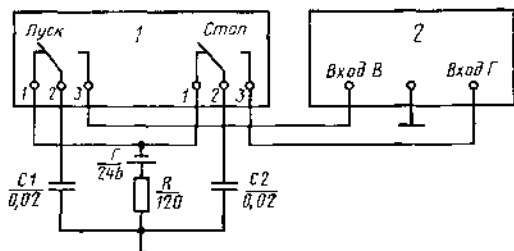
1—поверяемый прибор, 2—электронно-счетный частотомер, C1 и C2—электрические постоянные конденсаторы, R—постоянный резистор, G—источник постоянного тока
